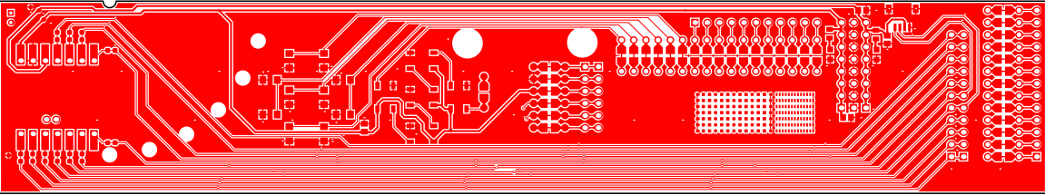
Top Layer (Scale 1:1.43)
